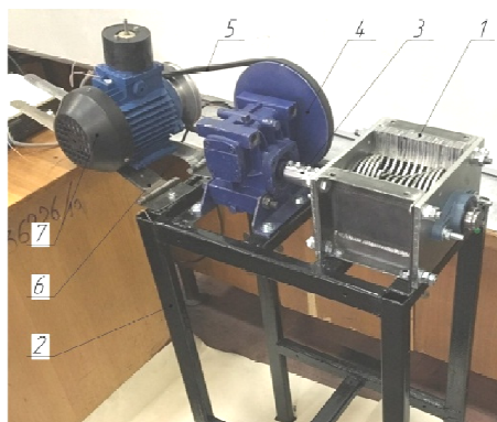
Рис. 3. Експериментальна установка шредера
